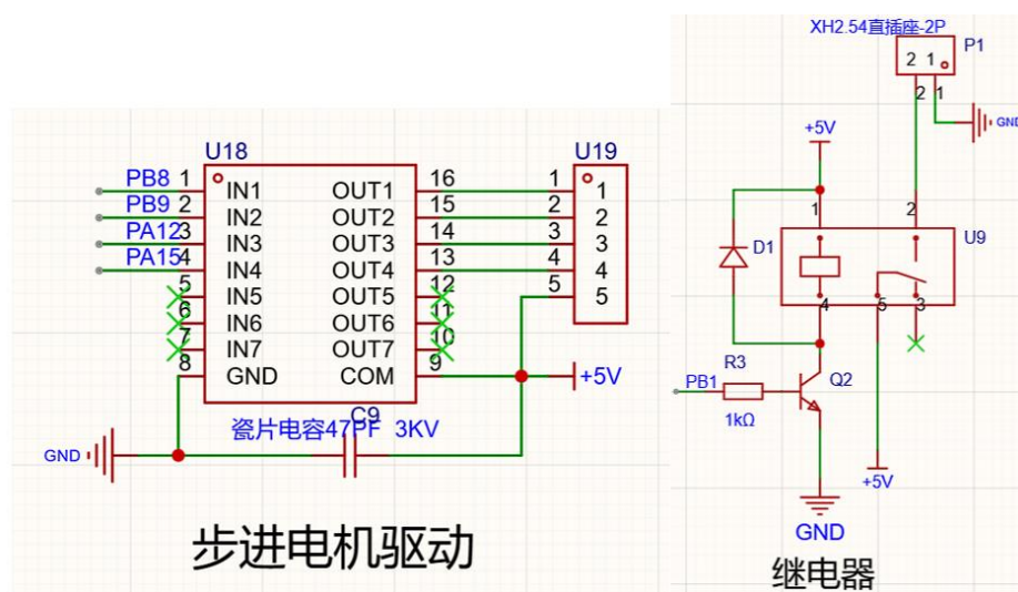
图 19 动作执行模块电路原理图
